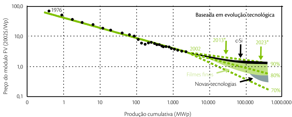
Figura 6: Curva de aprendizado para a energia solar fotovoltaica. Uma curva de aprendizado de 80% corresponde a uma redução de custos de 20% para cada dobro da produção acumulada.
