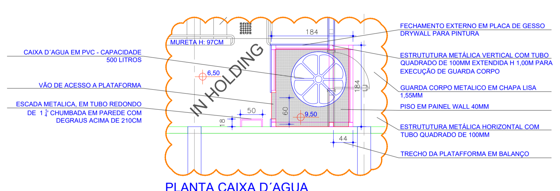
PLANTA CAIXA D'AGUA
