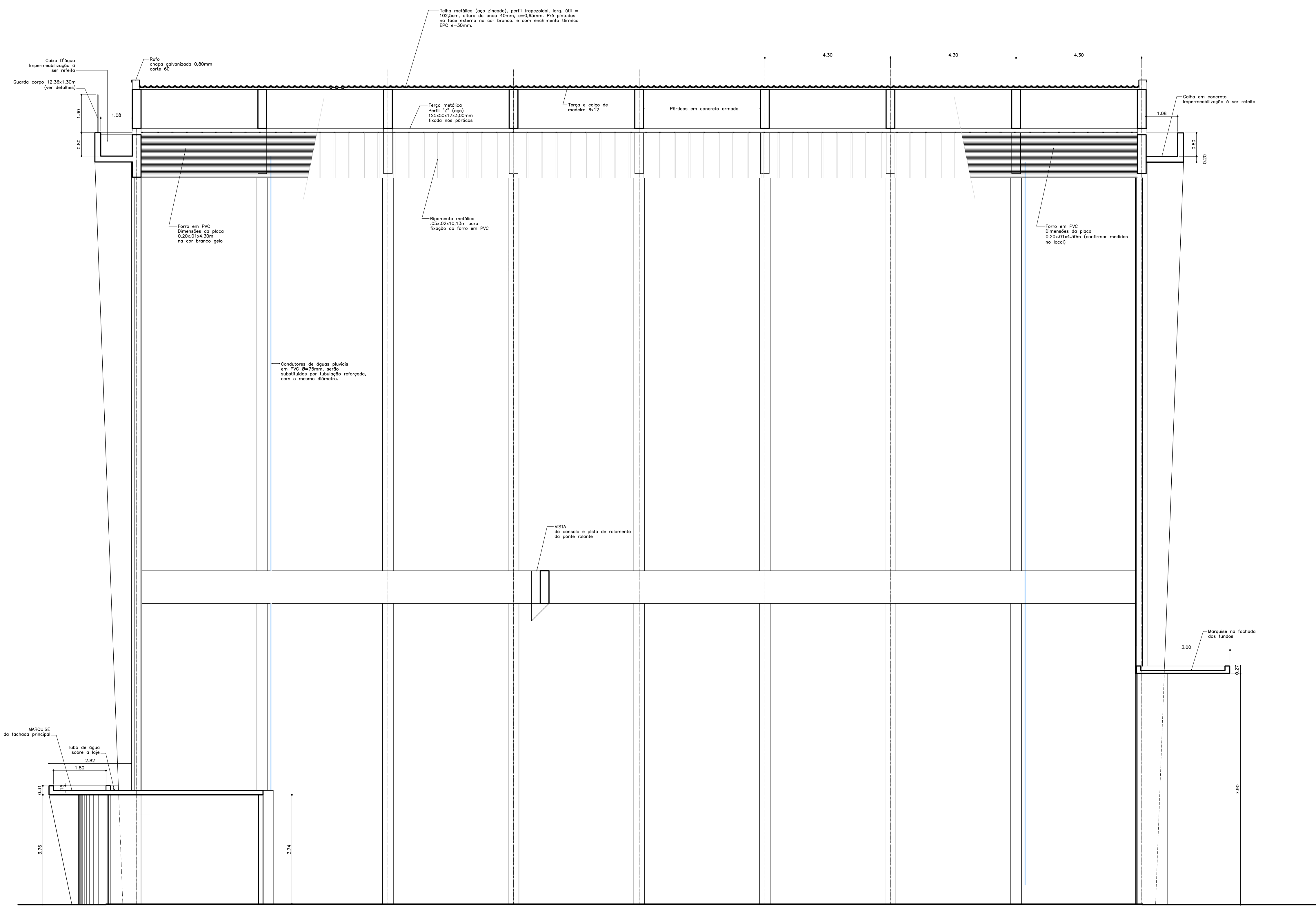
02 CORTE B-B ESC 1:75
