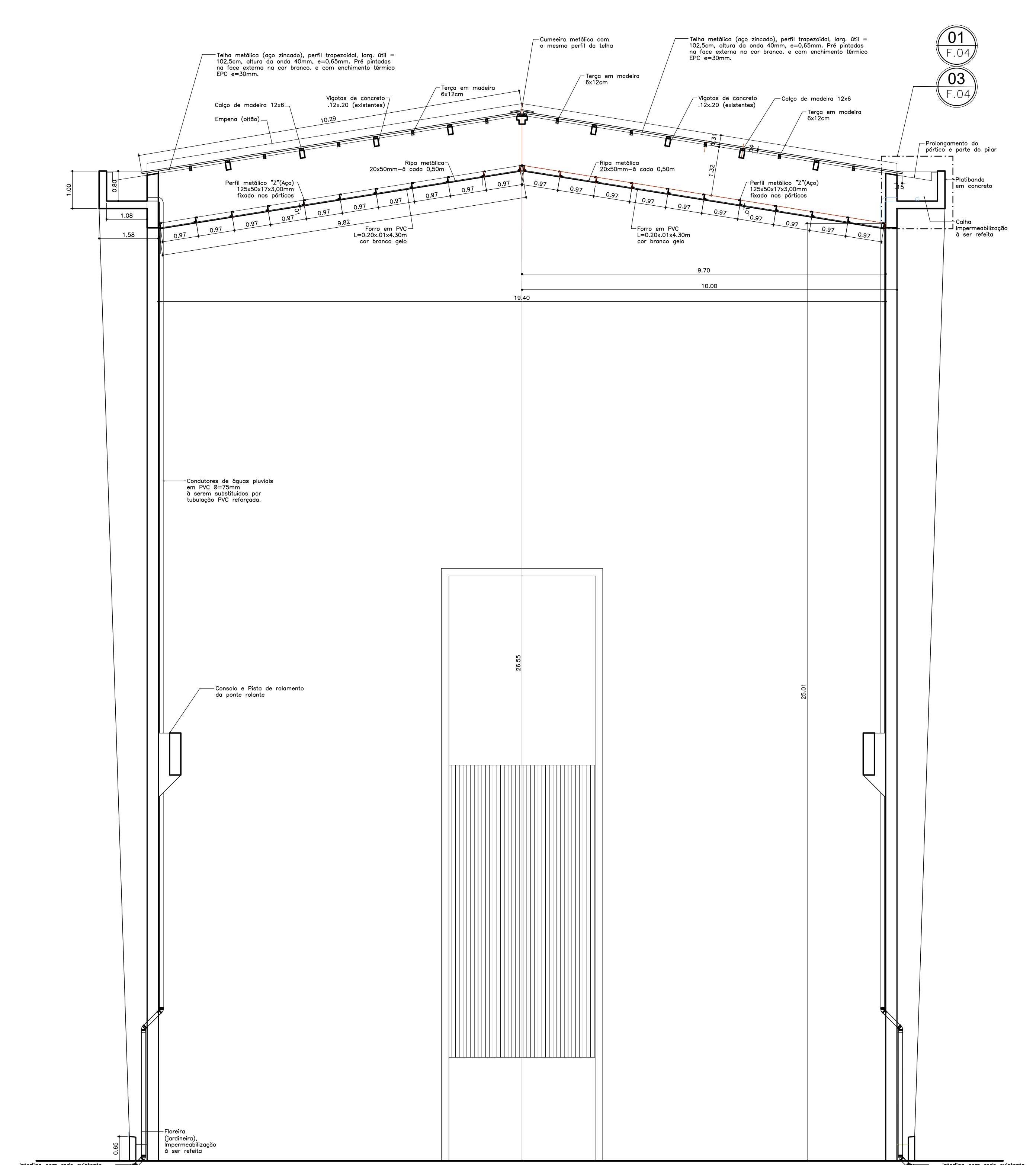
02 CORTE B-B ESC 1:75
